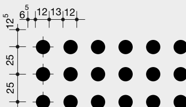
Регулярная круглая перфорация 12/25 R
