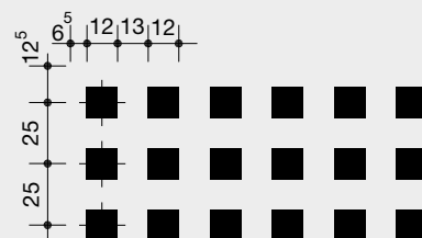
Регулярная квадратная перфорация 12/25 Q
