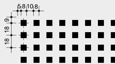
Регулярная квадратная перфорация 8/18 Q
