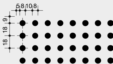
Регулярная круглая перфорация 8/18 R
